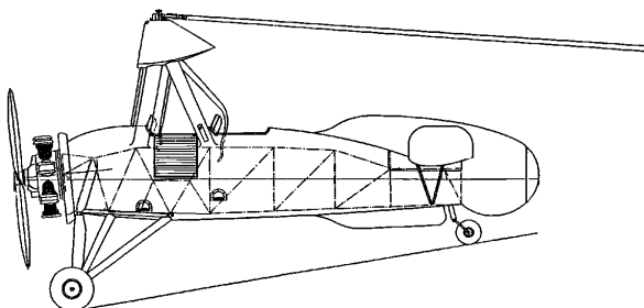
50.02.013 autogiro De La Cierva C30
